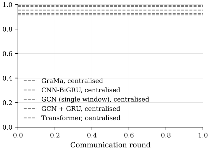
Test macro-F1
