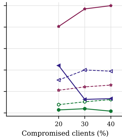
ALIE
