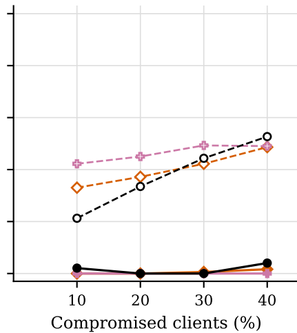
ALIE
