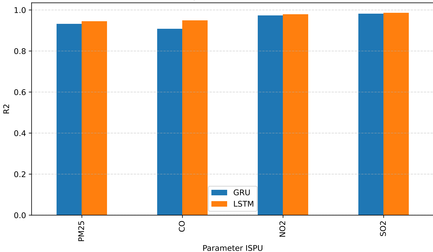
Perbandingan R2 GRU vs LSTM (ISPU)
