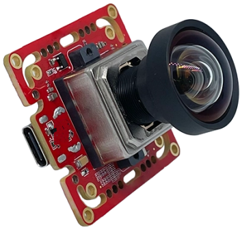
LYNX Lite-4K · USB 3.0 카메라
