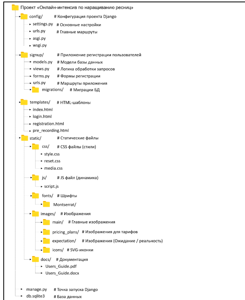
Рисунок 1. Структура сайта
