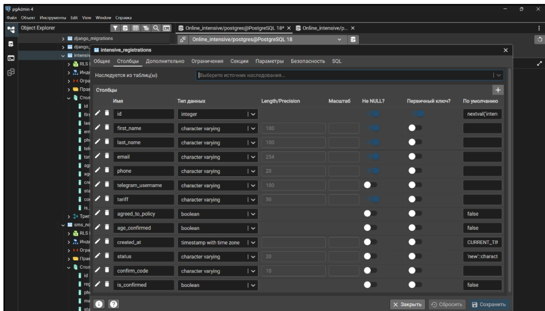
Рисунок 20. Структура таблицы «intensive_registrations» через графический интерфейс «pgAdmin 4»
