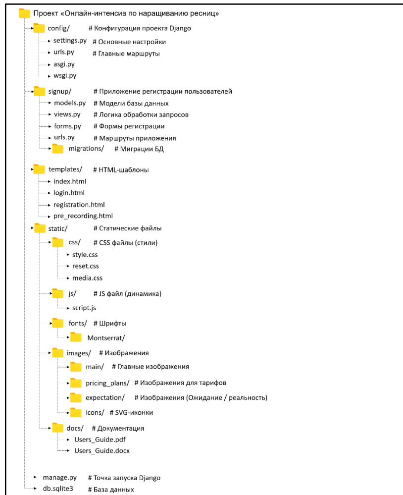
Рисунок 1. Структура сайта
