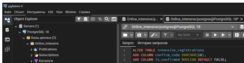
Рисунок 19. Расширение структуры таблицы с помощью команды Были добавлены дополнительные поля:
