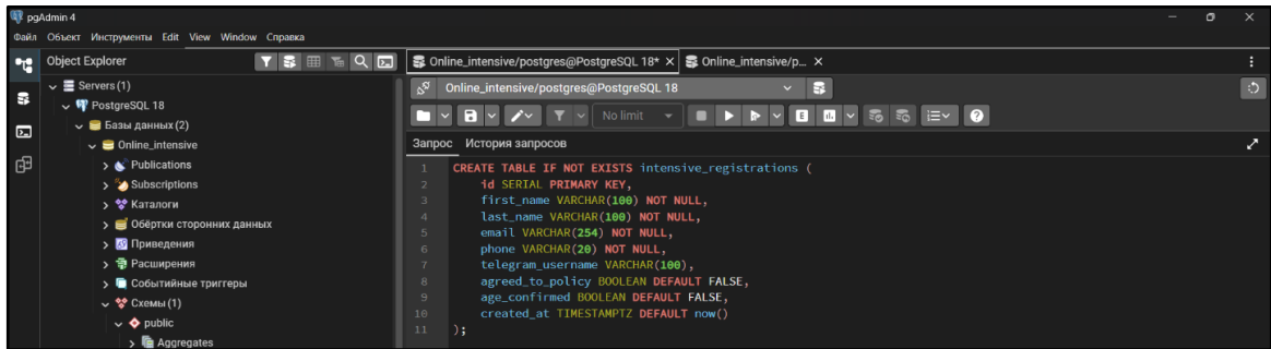
Рисунок 18. SQL-запрос создания таблицы «intensive_registrations»
