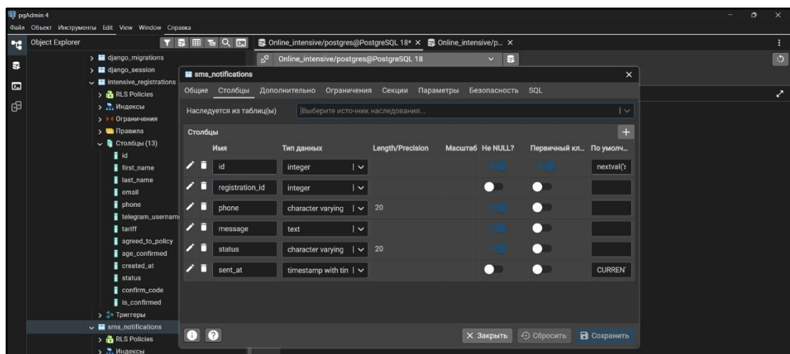
Рисунок 21. Структура таблицы «sms_notifications»
