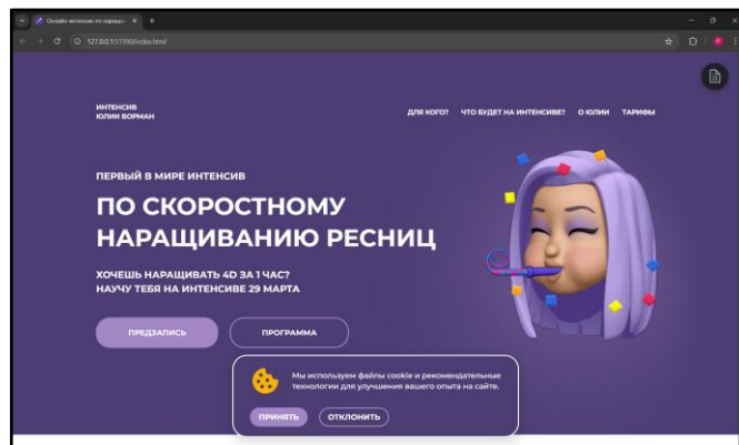
Рисунок 2. Главный экран
