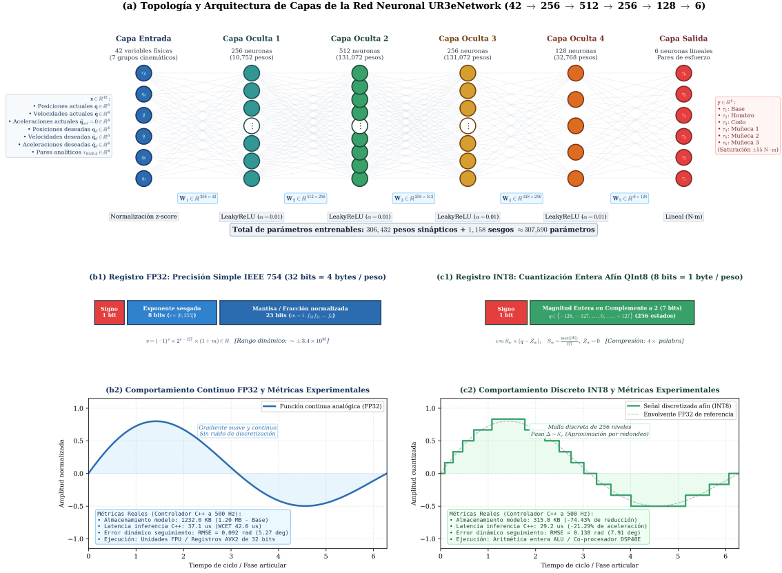
Figura 7: Diseño del módulo de compensación inteligente ( M_3 ): (a) Arquitectura y topología de capas del perceptrón multicapa UR3eNetwork (42 → 256 → 512 → 256 → 128 → 6); (b1, b2) Estructura del registro IEEE 754 de 32 bits y percepción de resolución continua en punto flotante FP32; (c1, c2) Formato de registro afín de 8 bits y percepción de malla discreta escalonada en enteros INT8 (QInt8), con resumen comparativo de recursos en tiempo real.
