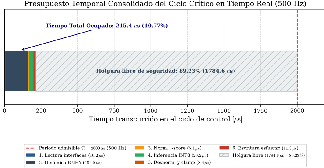
Figura 11: Presupuesto y distribución temporal del ciclo de control a 500 Hz ( T_s = 2000 \mu s): Desglose de latencias por subproceso dentro del bucle de control de par neuronal INT8 (215,4 \mu s de cómputo activo total) y margen determinista de holgura libre del 89,23 % (1784,6 \mu s).
