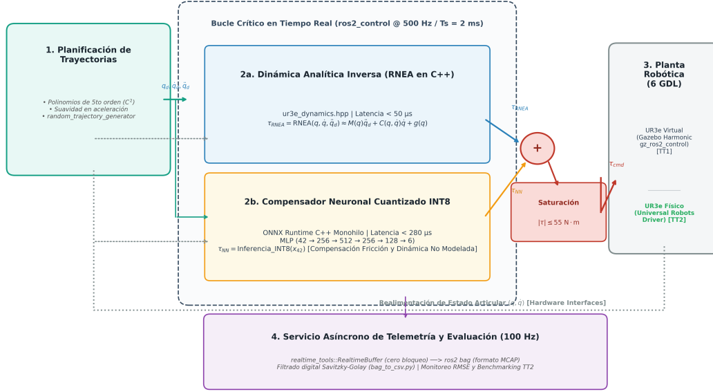
Figura 8: Diagrama de integración mecatrónica global: interconexión de nodos, buses en tiempo real y acoplamiento temporal de la arquitectura híbrida.
