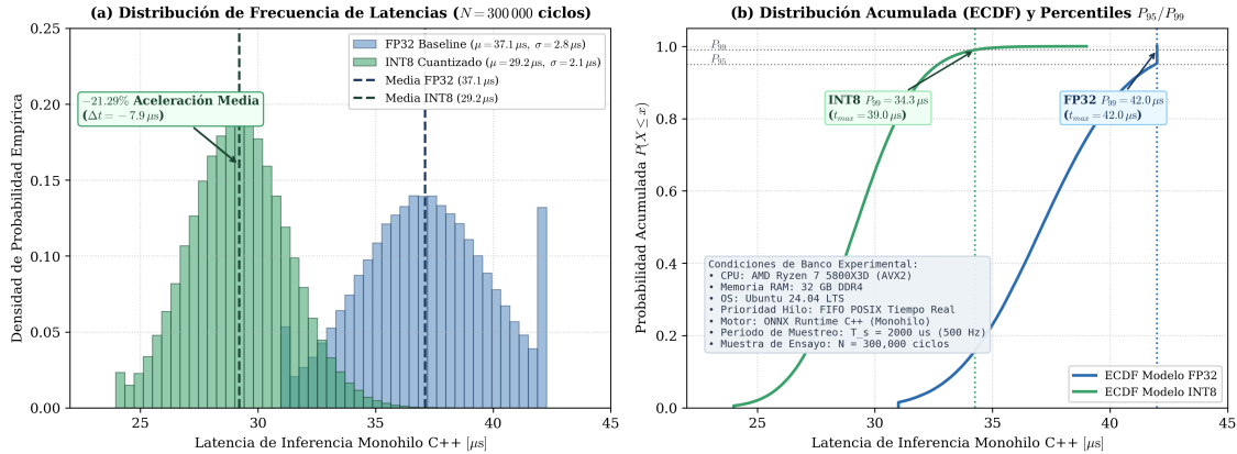
Figura 10: Distribución estadística empírica de la latencia de inferencia monohilo en C++ ( N = 300\,000 ciclos a 500 Hz): (a) Histograma de frecuencias y densidad para el modelo FP32 ( \mu = 37,1 \mu s) frente al modelo cuantizado INT8 ( \mu = 29,2 \mu s); (b) Función de distribución acumulada empírica (ECDF) con percentiles P_{95} , P_{99} y caso extremo t_{max} , evidenciando una cota inferior a 35 \mu s para el 99 % de los ciclos de control.
