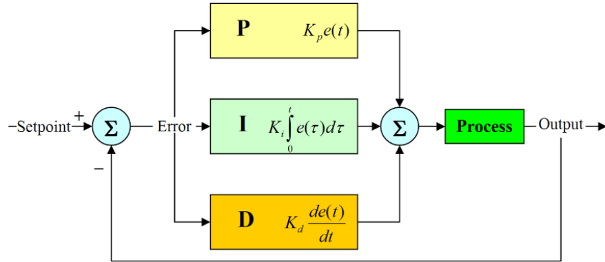
Figura 3: Diagrama simplificado de un control PID [16].
