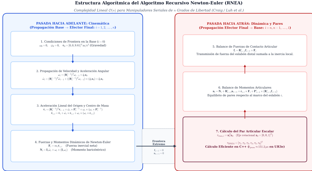
Figura 2: Diagrama de flujo del Algoritmo Recursivo de Newton-Euler (RNEA) bajo la convención Denavit-Hartenberg modificada (Craig): propagación cinemática hacia adelante ( i = 1 \dots n ) y balance cinético de fuerzas y momentos hacia atrás ( i = n \dots 1 ).
