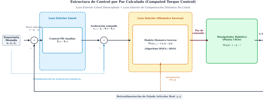
Figura 3: Diagrama de bloques del esquema de control por par calculado ( Computed Torque Control - CTC) con desacoplamiento no lineal de inercia \mathbf{M}(\mathbf{q}) , efectos centrífugos/Coriolis \mathbf{C}(\mathbf{q}, \dot{\mathbf{q}}) y gravedad \mathbf{g}(\mathbf{q}) .
