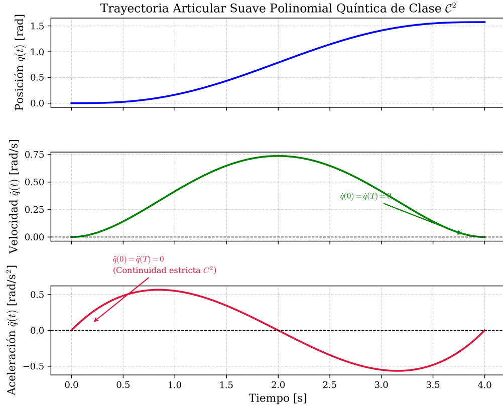
Figura 11: Perfiles cinemáticos suaves de posición, velocidad y aceleración articular generados mediante interpolación polinomial quíntica de clase C^2 , evidenciando derivadas continuas y nulas en los extremos temporales.
