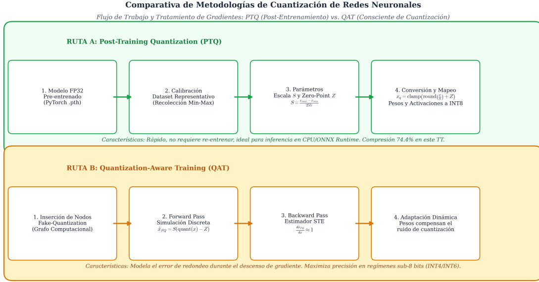
Figura 4: Comparativa de flujos metodológicos para la cuantización de redes neuronales: Ruta A ( Post-Training Quantization - PTQ) mediante calibración sobre grafo estático con métricas Min-Max, y Ruta B ( Quantization-Aware Training - QAT) con inserción de nodos Fake-Quantization y propagación de gradientes con el estimador STE.
