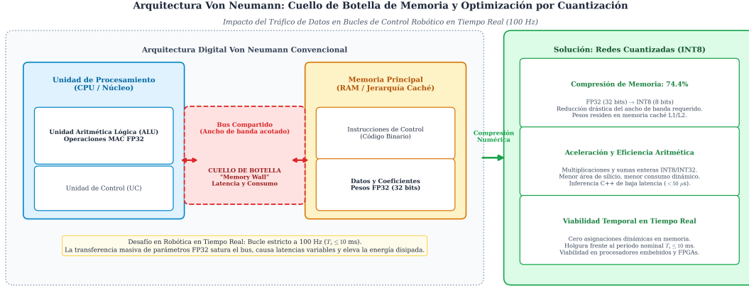
Figura 1: Cuello de botella de Von Neumann en la computación robótica convencional: latencia y costo computacional asociados a la transferencia masiva de datos en el bus CPU-Memoria ( Memory Wall ) frente al beneficio de la cuantización INT8 para la reducción de transferencias y la viabilidad de cálculo en lazos en tiempo real ( T_s \leq 10 ms).
