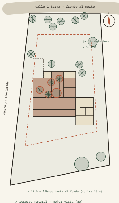
Lote 054 a escala (la barra mide 10 m). Línea roja punteada: retiros obligatorios.
