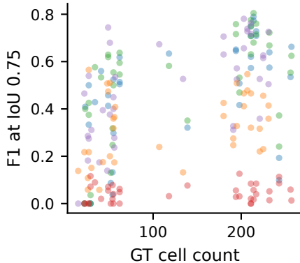
(b) F1 at IoU 0.75 ( r=0.33 , p=0.000 )
