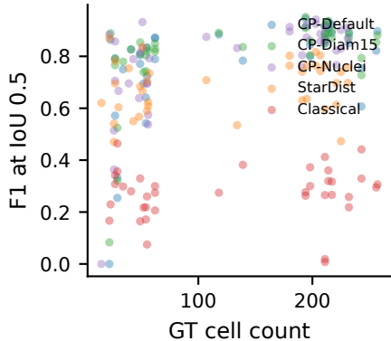
(a) F1 at IoU 0.5 ( r=0.29 , p=0.000 )
