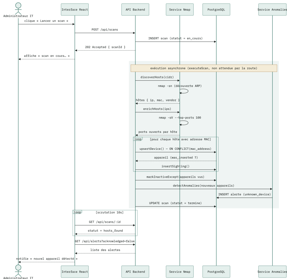
FIGURE 3.2 – Diagramme de séquence – exécution d'un scan et détection d'une anomalie
