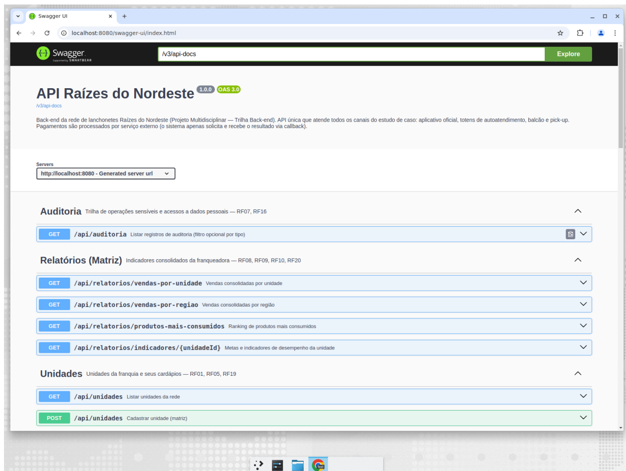
Figura 5: Swagger UI
