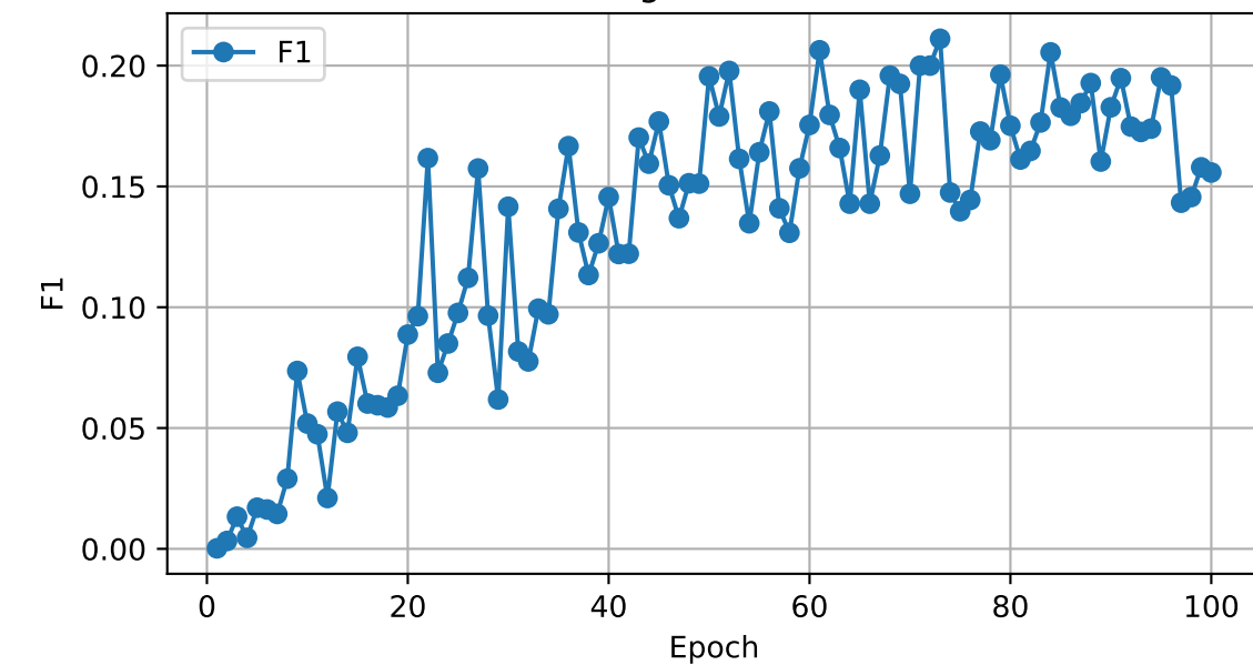
sigma8 - F1
