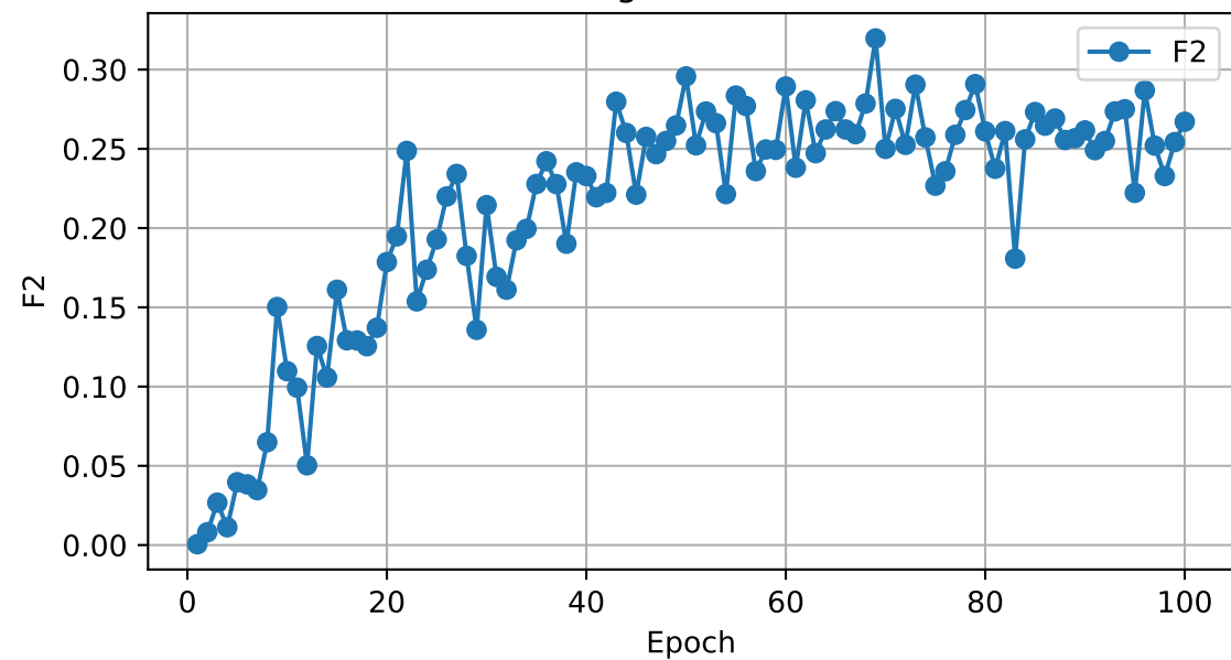
sigma8 - F2
