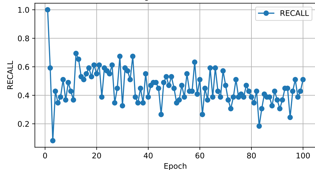
sigma8 - F2
