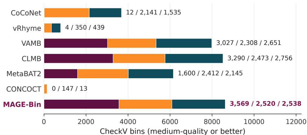
(e) Soil (metaFlye)
