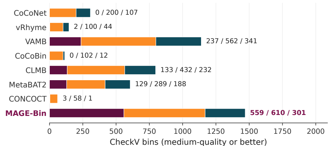
(d) IBD (metaFlye)
