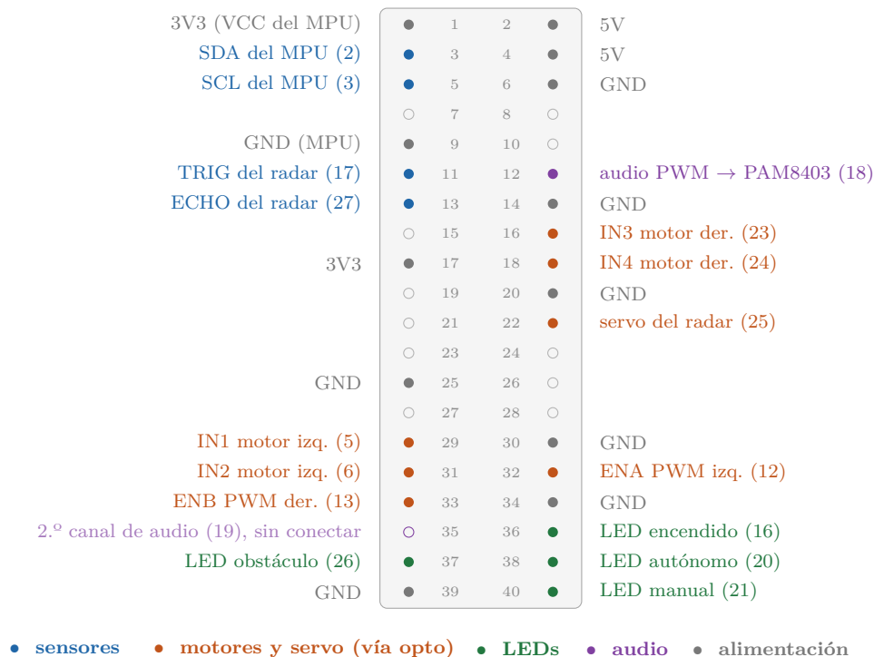
Figura 8: Conector de 40 pines. GPIO 12 y 13 son los canales PWM0/PWM1 del SoC: permiten migrar los motores a PWM por hardware sin recablear. Por eso el audio usa el otro par que admite audremap , GPIO 18/19. GPIO 2/3 son el bus I2C-1 del MPU-6050. GPIO 14/15 (UART) quedan libres para la consola serie de depuración.
