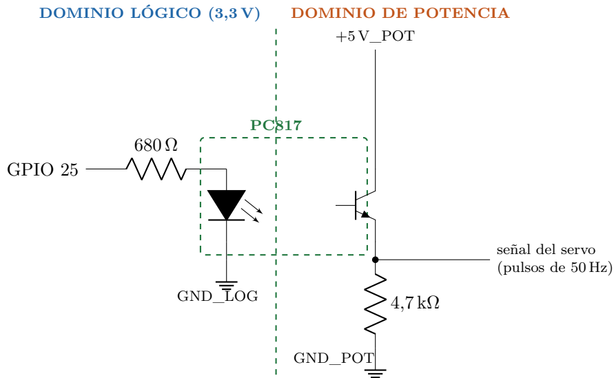
Figura 3: Canal del servo (7 de 7). Seguidor de emisor: la salida se toma del emisor, con una resistencia a GND_POT , y no invierte . Con emisor común, el GPIO en reposo —en el arranque, o con el servidor detenido— sería un nivel alto permanente que lleva al servo contra su tope.
