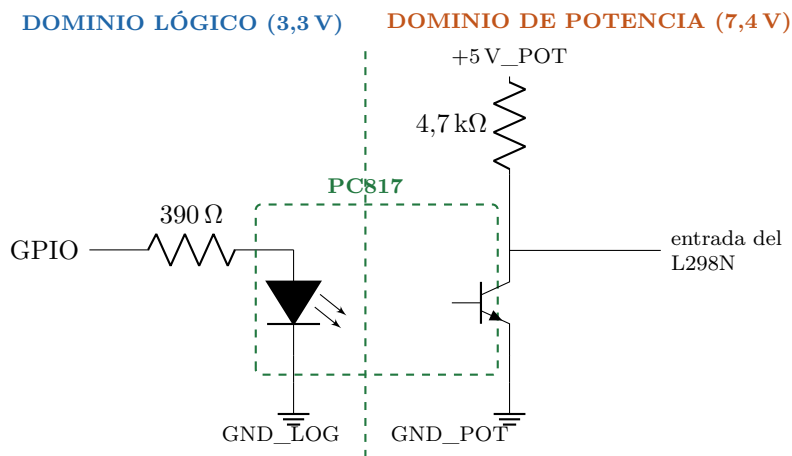
Figura 2: Canal de aislamiento con PC817 (6 de 7: las señales del L298N). Emisor común: el fototransistor conduce cuando el LED enciende, de modo que la señal sale invertida . Se compensa en lib/lib_motors.c .
