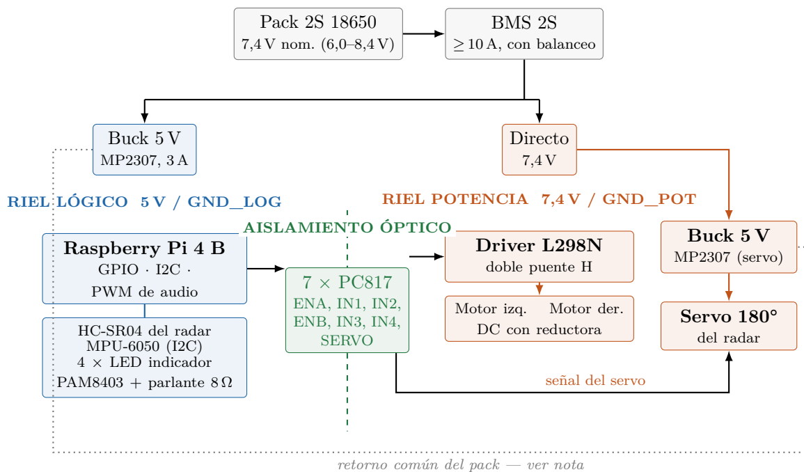
Figura 1: Arquitectura de hardware: fuente única, dos rieles regulados por separado, el servo del radar con su propio regulador en el riel de potencia y barrera óptica en las siete señales de control.
