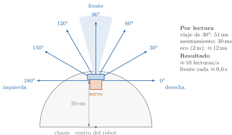
Figura 4: Radar visto desde arriba. El servo se detiene cada 30° en vaivén (0 → 180 → 0) y en cada parada se dispara el HC-SR04, cuyo cono de \sim 15^\circ de semiapertura (sombreado a 90°) solapa con el de las lecturas vecinas. Cada lectura frontal con eco actualiza el tiempo antes de chocar.
