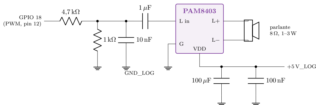
Figura 7: Salida de audio. El divisor baja el PWM de 3,3 V a unos 0,2 V RMS y, con los 10 nF, forma un pasabajos de 19 kHz que quita la portadora; con los 24 dB del PAM8403 da \approx 1,3 W en 8 \Omega . El parlante va entre L+ y L-: las salidas son en puente y ninguna va a tierra. El amplificador se alimenta del riel lógico, lejos del ruido de los motores; el volumen se controla por software con amixer .
