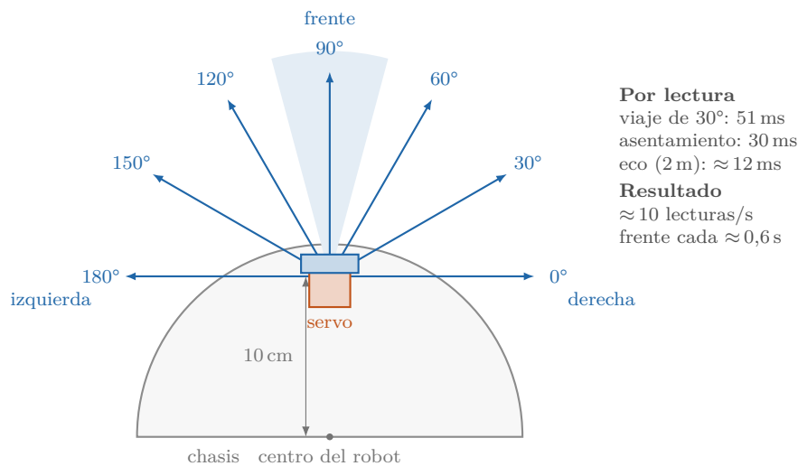
Figura 4: Radar visto desde arriba. El servo se detiene cada 30° en vaivén (0 → 180 → 0) y en cada parada se dispara el HC-SR04, cuyo cono de ~15° de semiapertura (sombreado a 90°) solapa con el de las lecturas vecinas. Cada lectura frontal con eco actualiza el tiempo antes de chocar.
