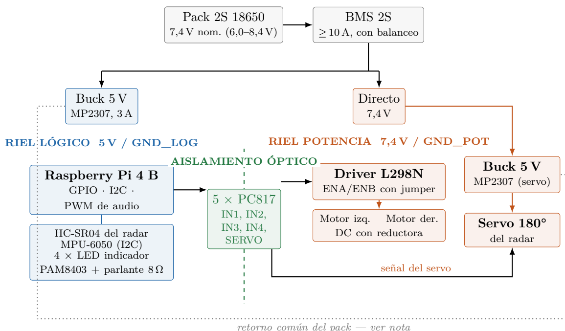
Figura 1: Arquitectura de hardware: fuente única, dos rieles regulados por separado, el servo del radar con su propio regulador en el riel de potencia y barrera óptica en las cinco señales de control.
