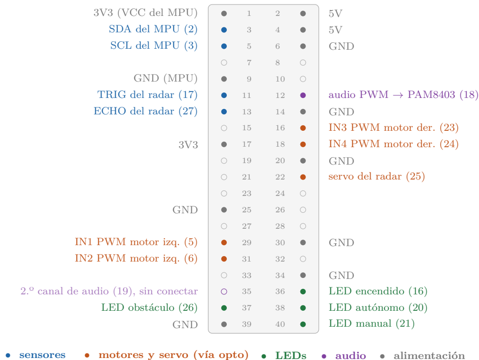
Figura 8: Conector de 40 pines. La PWM de los motores va sobre las entradas del L298N (GPIO 5, 6, 23 y 24); pigpiod la genera por DMA en cualquier GPIO. GPIO 12 y 13, que llevaban ENA/ENB, quedan libres. El audio sale por GPIO 18 con audremap ; GPIO 2/3 son el bus I2C-1 del MPU-6050; GPIO 14/15 (UART) quedan libres para la consola serie.
