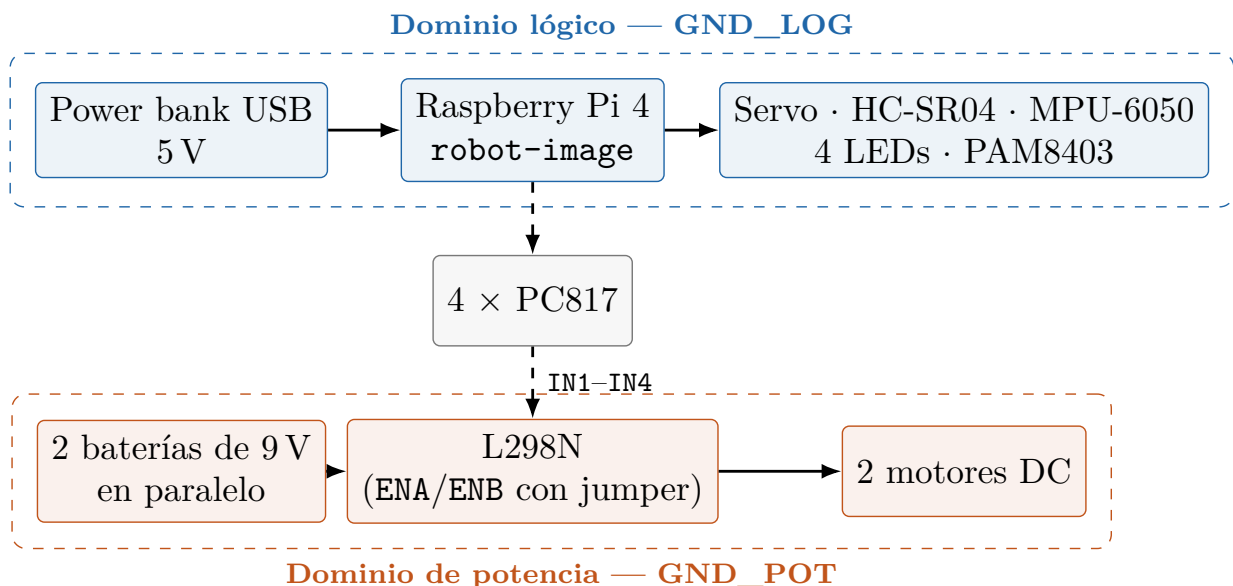
Figura 1: Arquitectura de hardware. Las líneas punteadas son señales que cruzan la barrera óptica. Los esquemas eléctricos completos están en hardware-diagramas.pdf .
