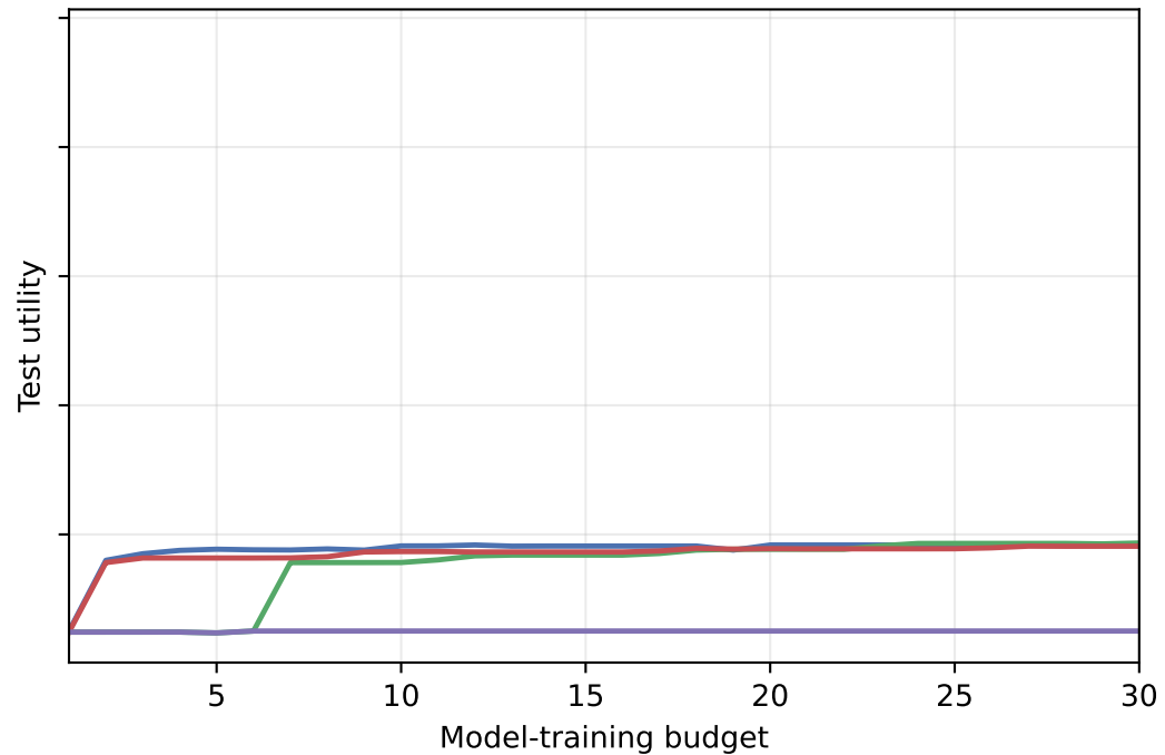
Classification — Data-Bandit — Data-All — Data-Alt — AutoML
