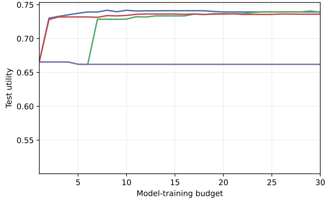
Classification — Data-Bandit — Data-All — Data-Alt — AutoML
