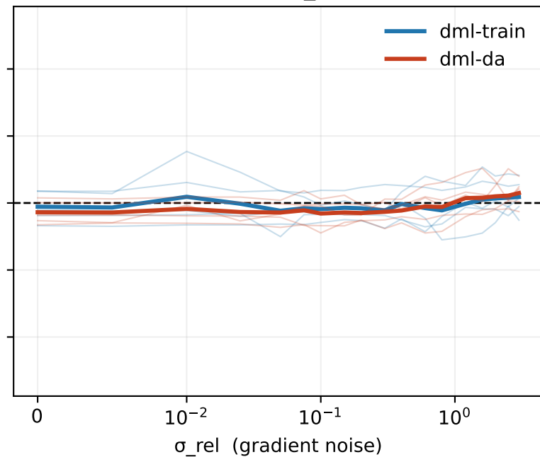
region = far_extrap
