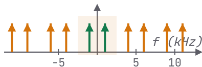
f_e = 5 \text{ kHz} : la bande gardée contient \pm 1 \text{ kHz} (vert)
