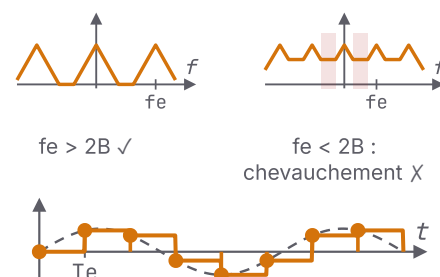
BOZ : paliers de durée T_e
