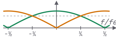
Ex. 2 passe-bas (vert) · Ex. 3 passe-haut (orange) · se croisent à 0,71 en fe/4
