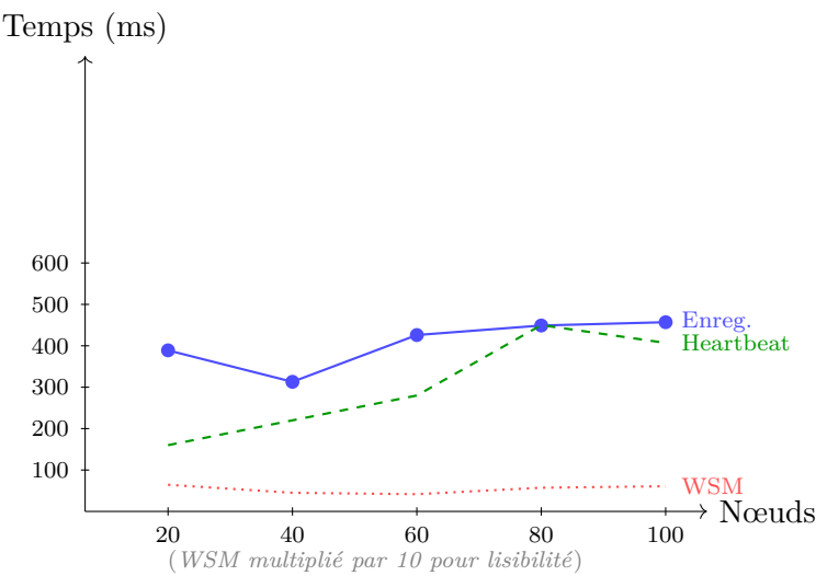
FIGURE 4.3 – Temps de réponse moyens en fonction du nombre de nœuds simulés.
