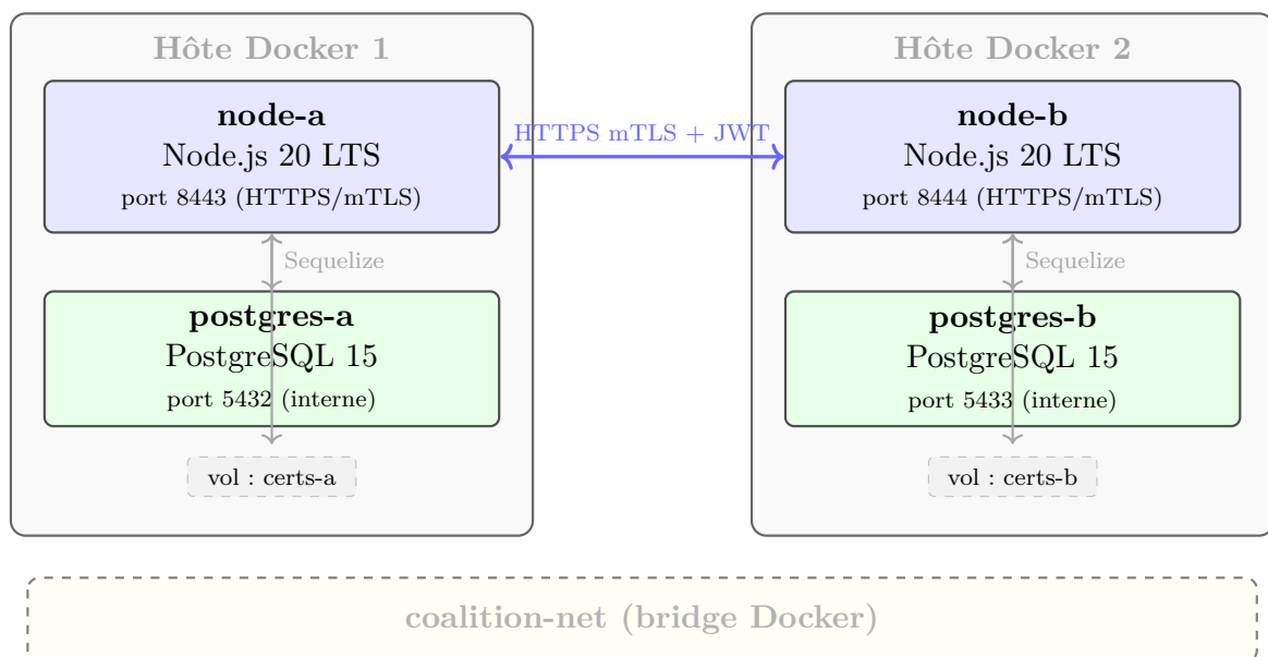
FIGURE 4.2 – Diagramme de déploiement : coalition à deux nœuds avec Docker.
