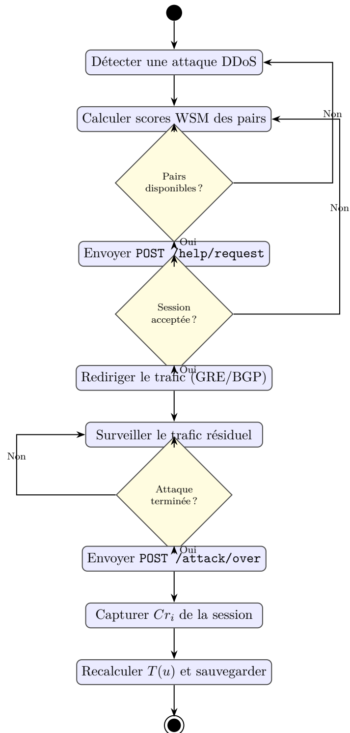
FIGURE 3.7 – Diagramme d'activités d'une session de mitigation collaborative.
