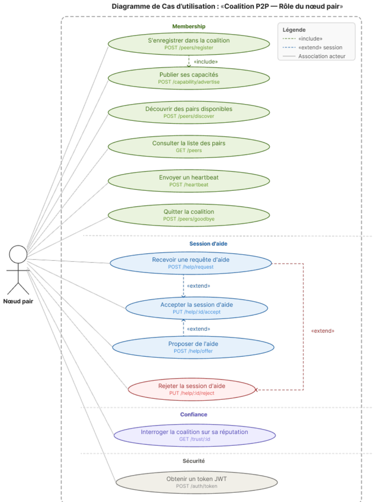
Figure 3.4 – Diagramme de cas d'utilisation : Rôle du nœud pair dans la coalition (12 cas d'usage).
