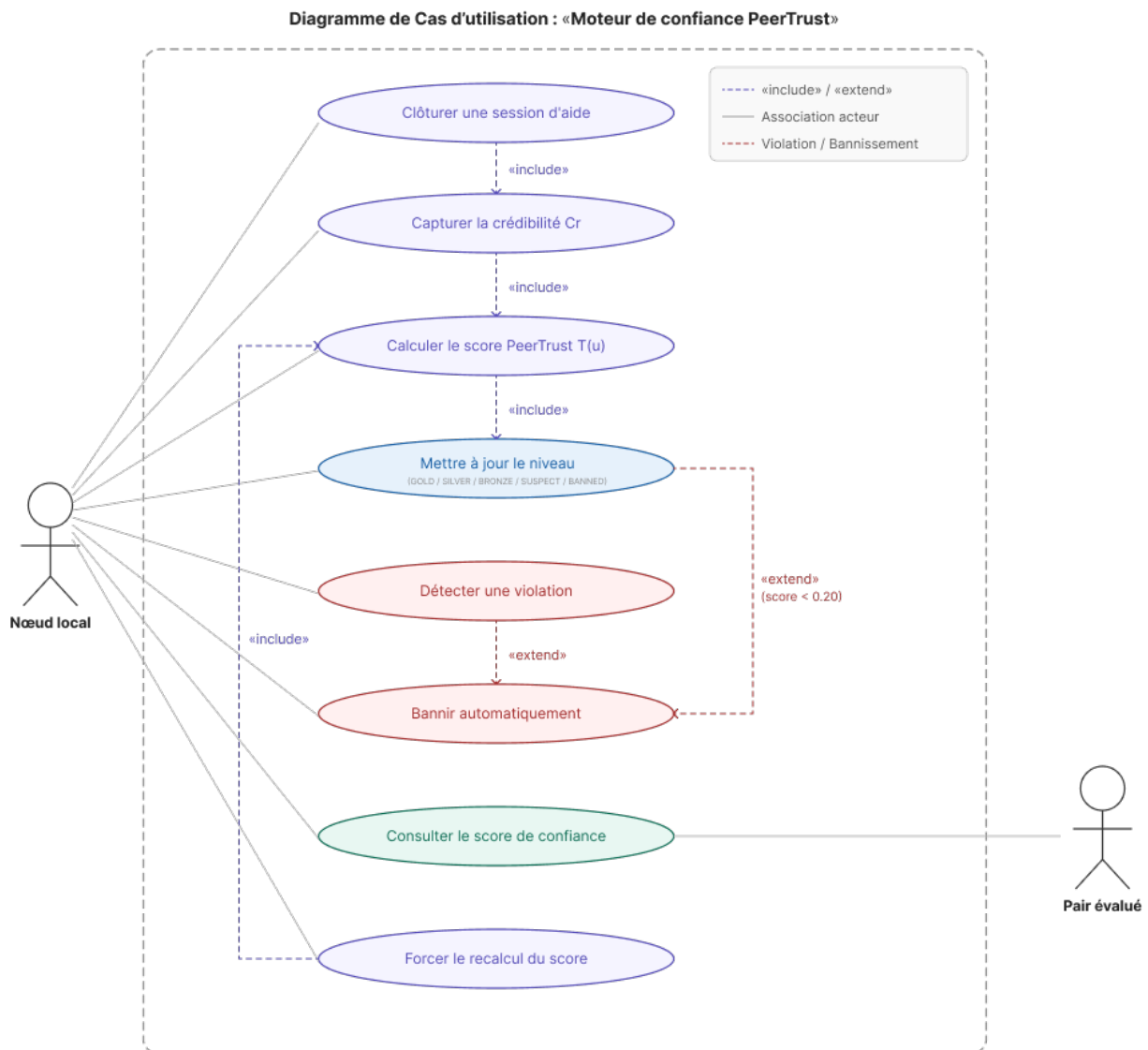
Figure 3.3 – Diagramme de cas d'utilisation : Moteur de confiance PeerTrust.
