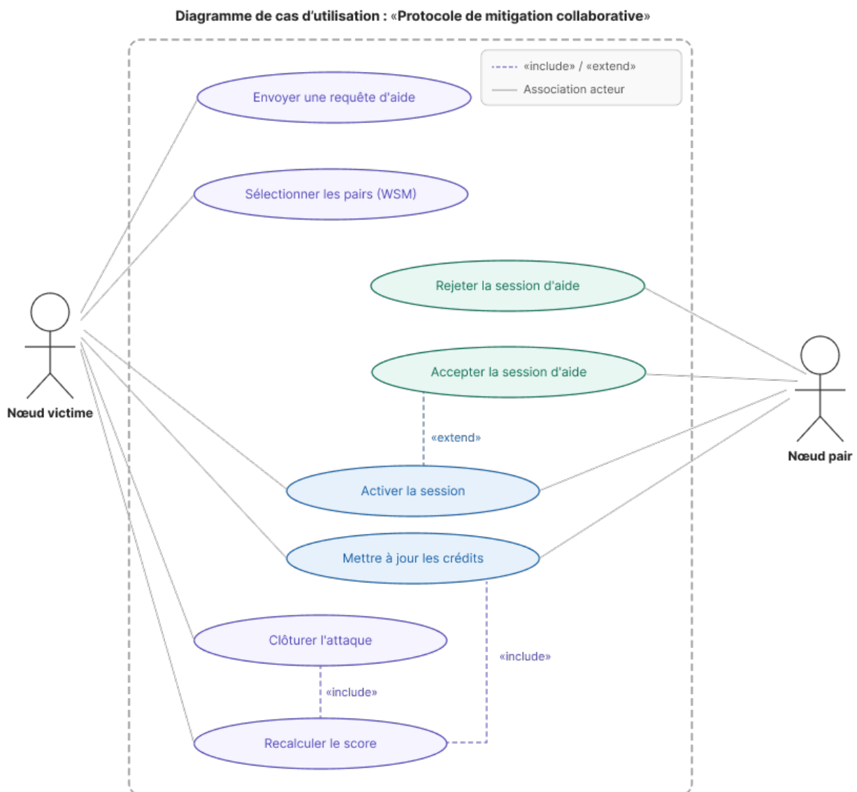
Figure 3.2 – Diagramme de cas d'utilisation : Protocole de mitigation collaborative.
