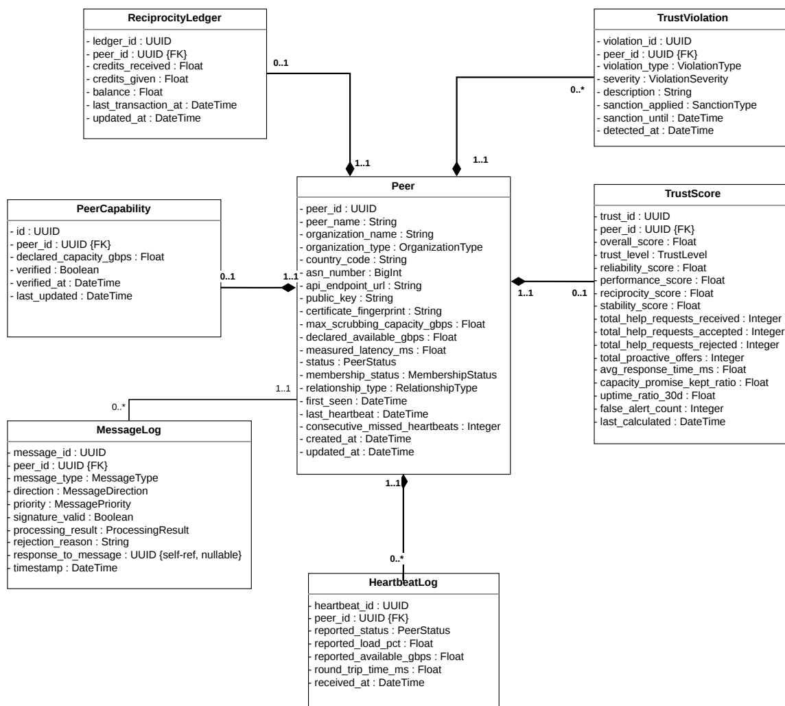
Figure 3.7 – Diagramme de classes — Gestion des pairs et de la confiance.
