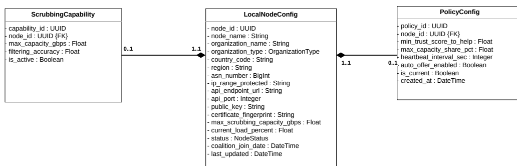
Figure 3.6 – Diagramme de classes — Configuration du nœud local.
