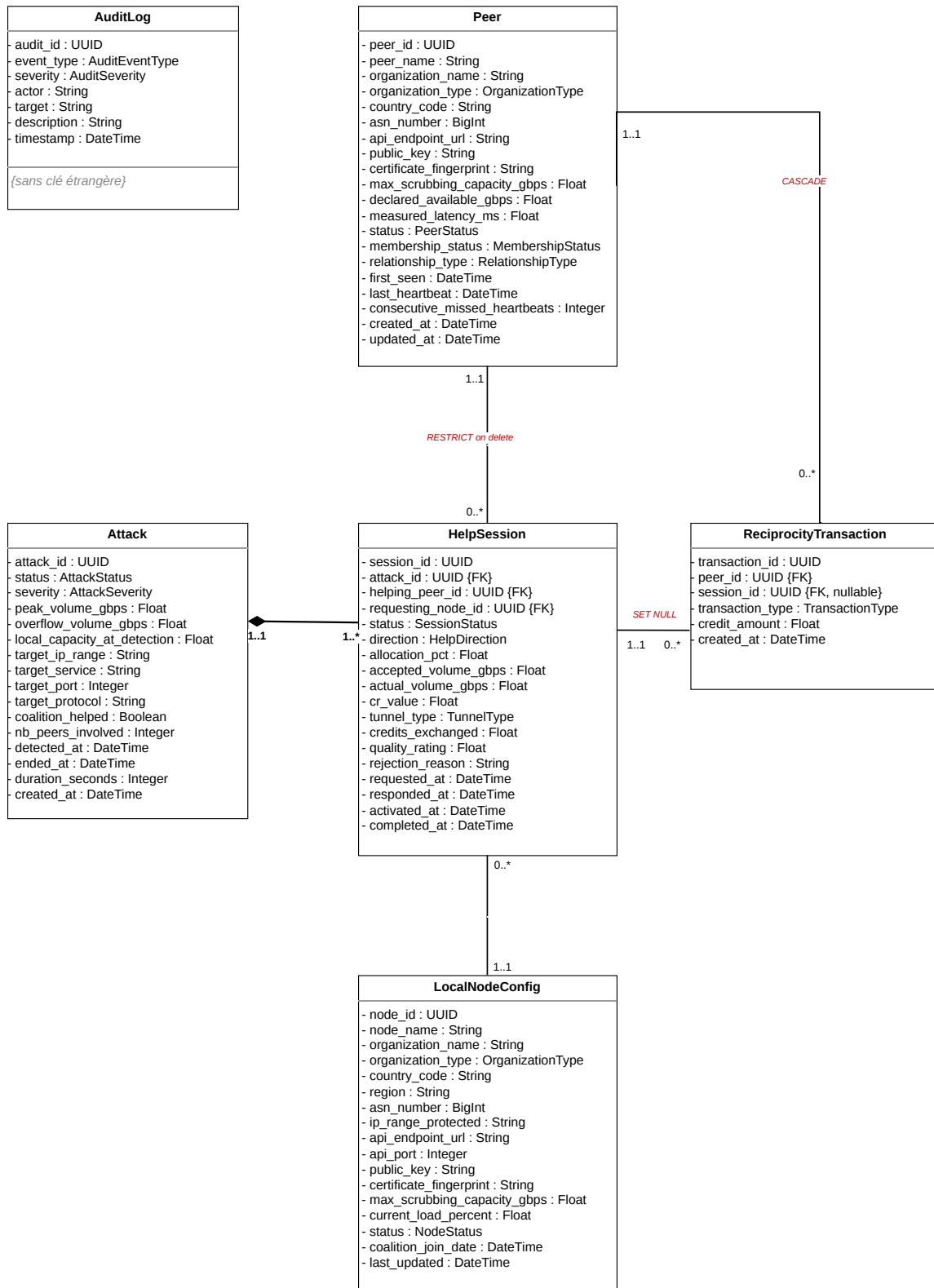
Figure 3.8 – Diagramme de classes — Sessions de mitigation et traçabilité.
