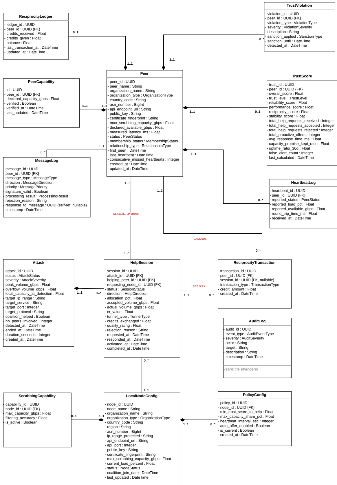
Figure 3.5 – Vue globale du diagramme de classes — les quatorze entités du système.
