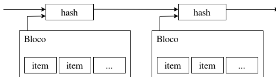
Figura 3 – Funcionamento do serviço de timestamp.
