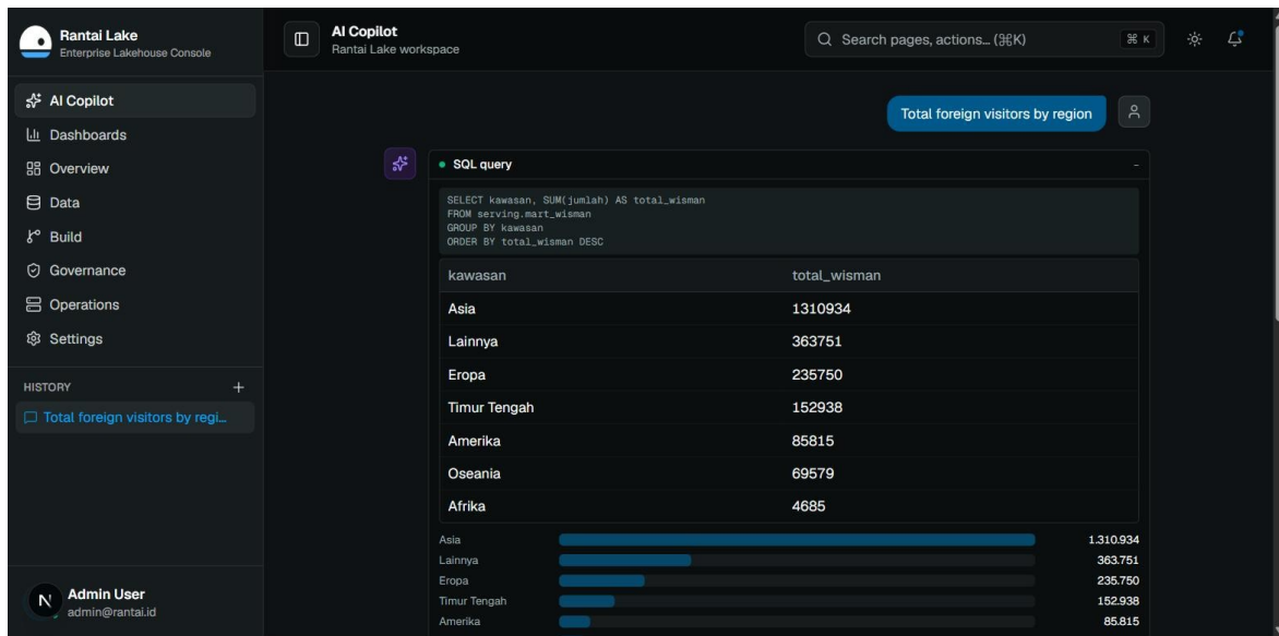
Gambar 5. Asisten data (AI Copilot) — pertanyaan bahasa sehari-hari dijawab dengan kueri yang ditampilkan terbuka beserta hasilnya.
