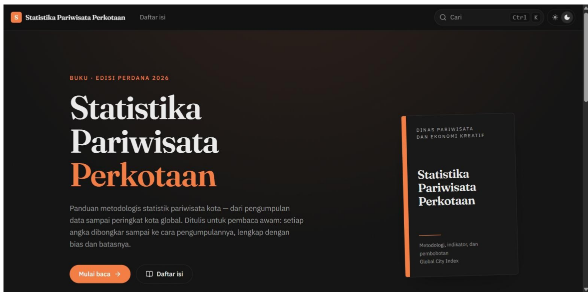
Gambar 9. Buku “Statistika Pariwisata Perkotaan” sebagai dokumentasi metodologi.
