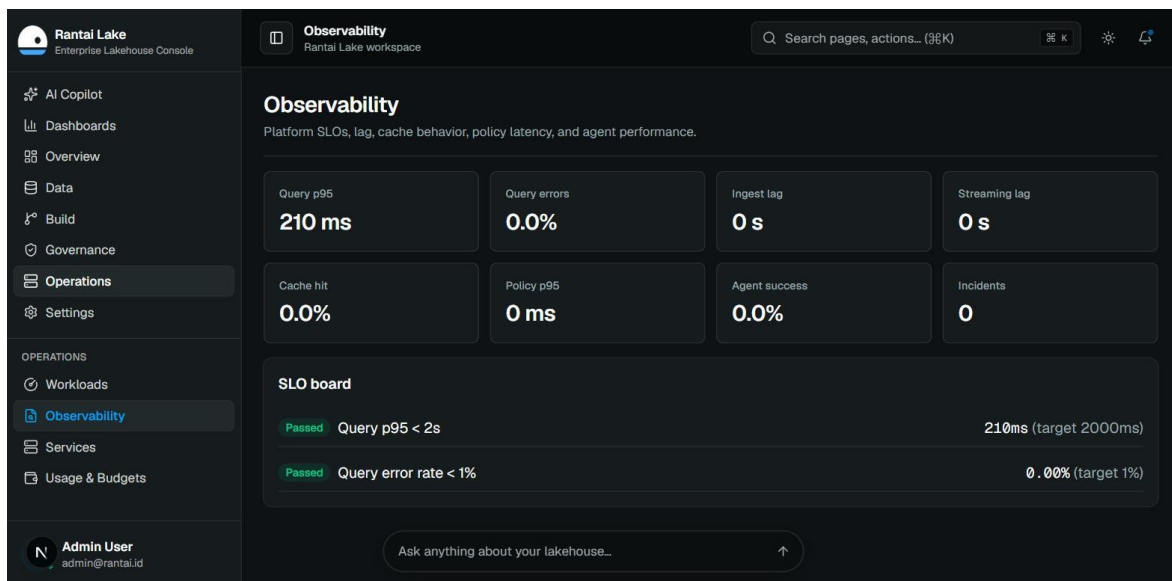
Gambar 2. Pemantauan kinerja — waktu respons kueri persentil-95 210 ms, kesalahan kueri 0%, tanpa insiden.
