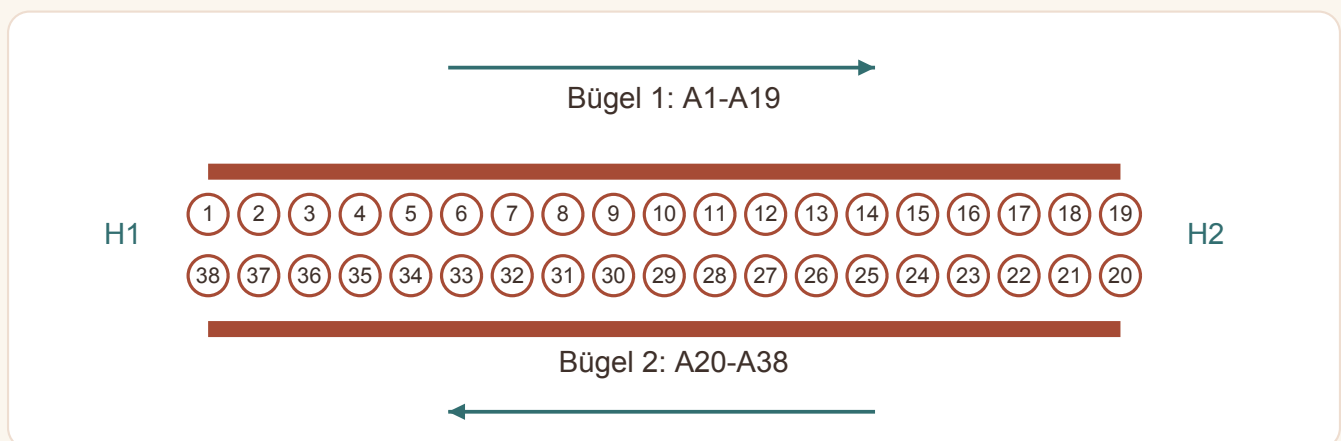
F12 | Neu nummerierte Öffnung: 19 Maschen pro Bügel; Gelenklücken H1/H2. Diagramm.
