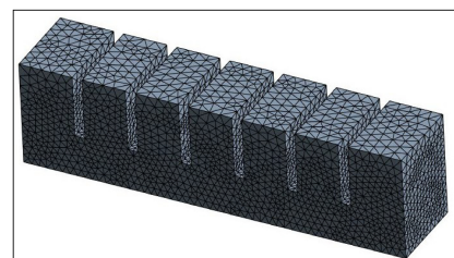
(b) Représentation du maillage du doigt [8]
