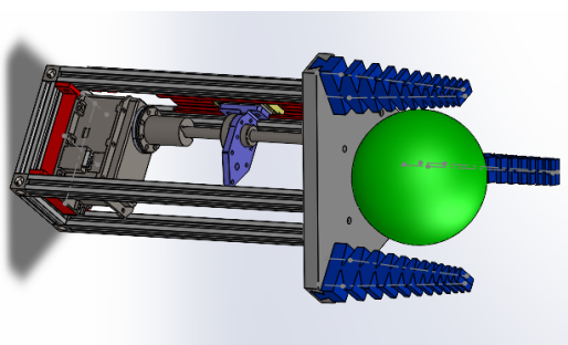
(a) Pince assemblée sur SolidWorks
