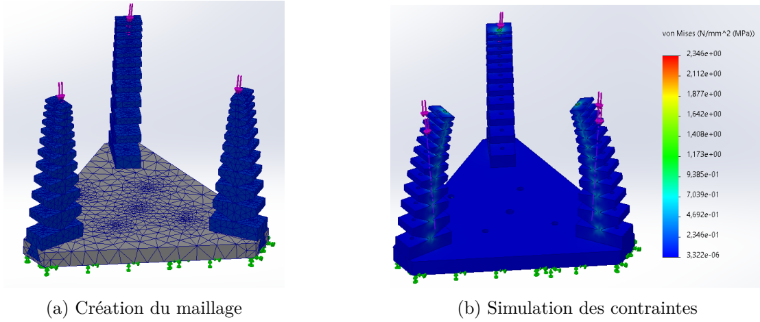
FIGURE 4.2 – Exécution de la simulation par éléments finis
