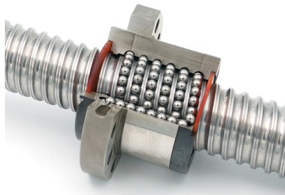
FIGURE 2.3 – Illustration en coupe d'une vis à billes [6]
