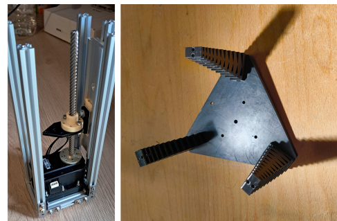
(b) Pièces imprimées et montage du support en MAKERBEAM
