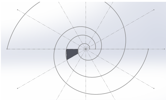
(a) Esquisse de l'étoile pour discrétiser la spirale, et extrusion de la moitié de la première phalange à l'aide des lignes construites
