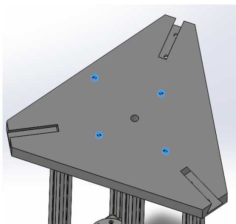
(a) 4 trous de diamètre 4,3 mm percés dans la base pour fixer les 4 barres (en bleu)
