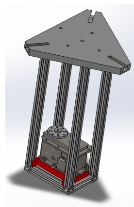
(b) Support moteur en MAKERBEAM, avec la pièce pour y fixer le moteur (en rouge)
