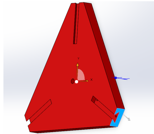
(b) Extrudage en queue de hareng de la même taille que celle du doigt, mais avec un jeu de 0.3 mm
