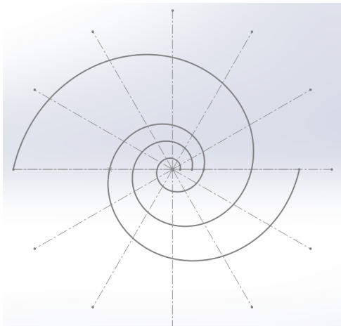
(a) Esquisse de l'étoile au centre du repère, pour discrétiser la spirale
