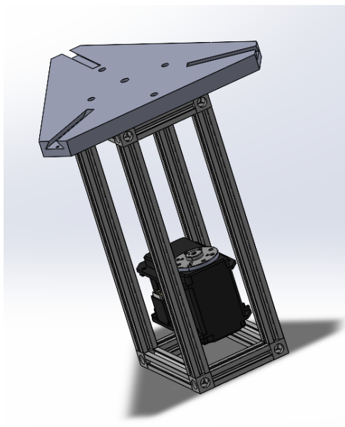
(a) Support moteur en MAKERBEAM
