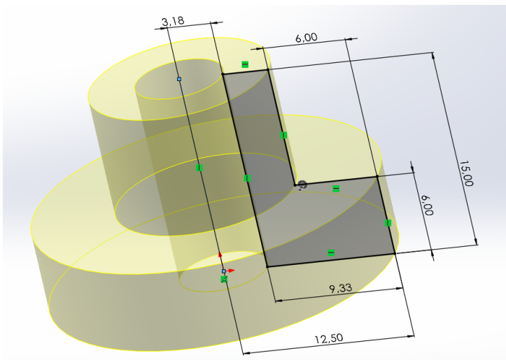
(a) Esquisse et bossage avec révolution
