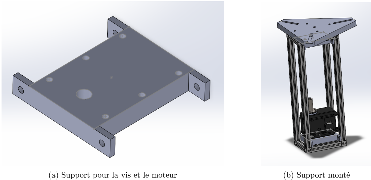
FIGURE III.13 – Conception du support du moteur
