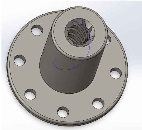
(a) Pièce attachée au moteur et vissée sur la vis mère
