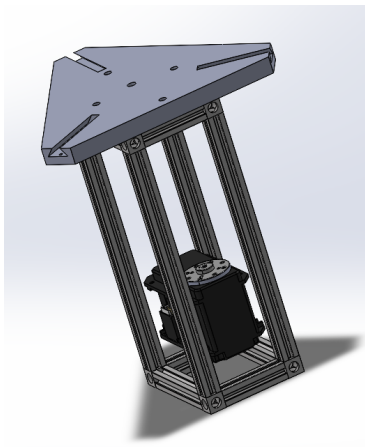
(a) Support moteur en MA-KERBEAM
