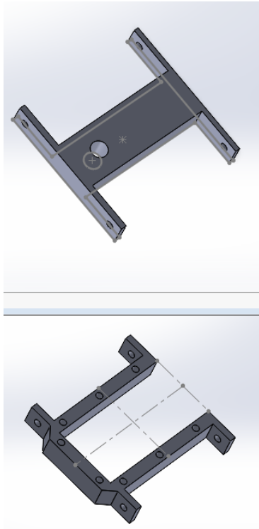
(a) Pièces de fixation pour la vis et le moteur
