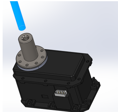
(b) Attache pour la vis mère et le moteur
