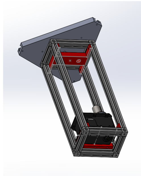
(b) Support assemblé avec les pièces de fixation (en rouge)
