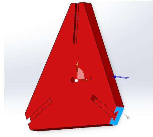
(b) Enlèvement de matière en queue de hareng de la même taille que celle du doigt, mais avec un jeu de 0.3 mm
