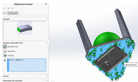
(a) Condition limite d'encastrement sur la base
