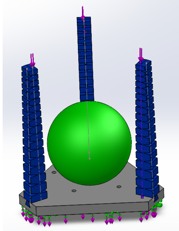
(b) Simulation des forces (en violet) engendrées par les câbles sur les doigts
