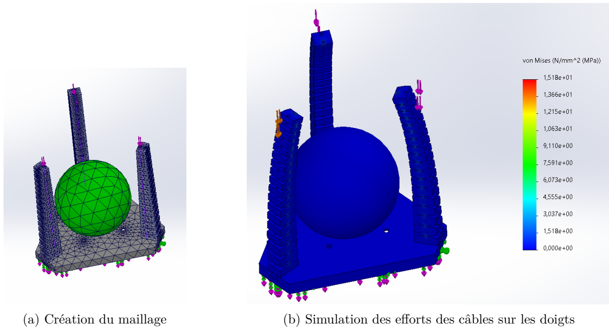
FIGURE IV.2 – Exécution de la simulation
