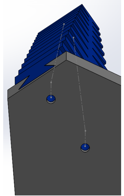
(b) Trous dans la base pour faire passer les câbles dans les doigts
