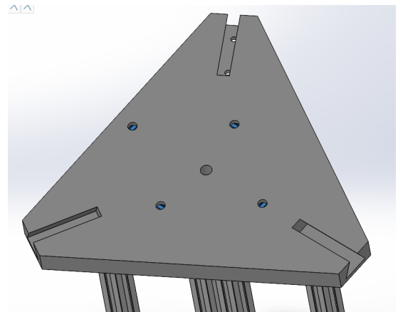
(b) 4 trous de diamètre 4 mm percés dans la base pour fixer les 4 barres (en bleu)
