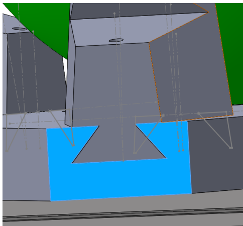
(a) Encastrement du doigt dans la base
