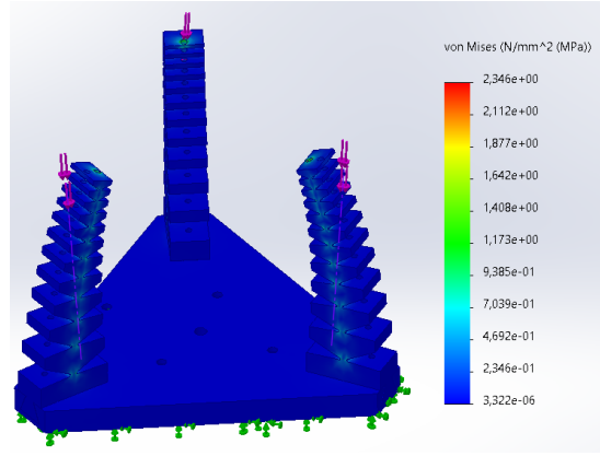
(b) Simulation des efforts des câbles sur les doigts
