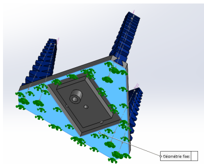
(a) Condition limite d'encastrement sur la base
