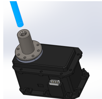
(b) Accouplement pour la vis mère (en bleue) et le moteur
