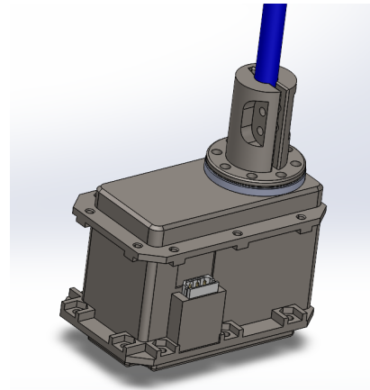
(b) Accouplement entre la vis mère (en bleue) et le moteur par le biais du dispositif de serrage
