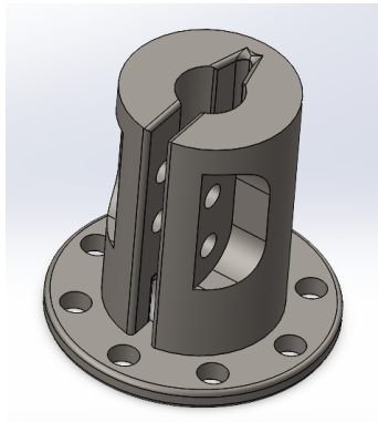
(a) Dispositif de serrage entre la vis et le moteur, pour transmettre le couple
