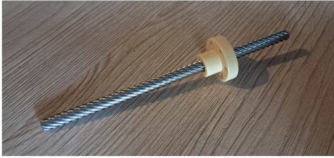
(a) Notre vis mère de la marque Igus en acier trempé, permettant un très faible frottement
