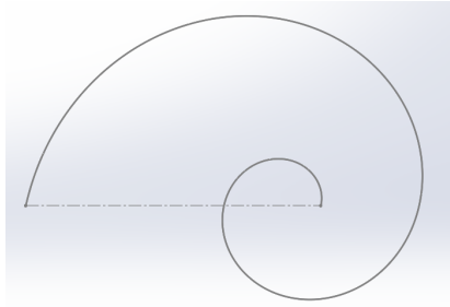
(a) Esquisse de la spirale centrale, d'équation r_c = a_c e^{b_c \theta} avec \theta \in [0, 3\pi]
