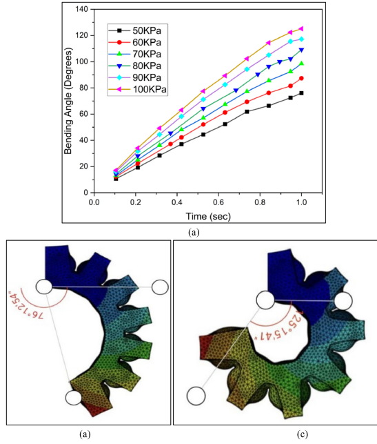
(a) Angle parcouru suivant la pression exercée (en haut), et effecteur pour une pression de 50 kPa et 100 kPa.
