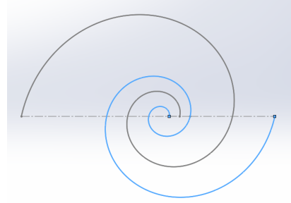
(b) Esquisse de la spirale qui enveloppe le doigt (en bleue), d'équation r = \frac{2 \cdot r_c(\theta)}{1 + e^{2\pi b}} avec \theta \in [0, 4\pi]
