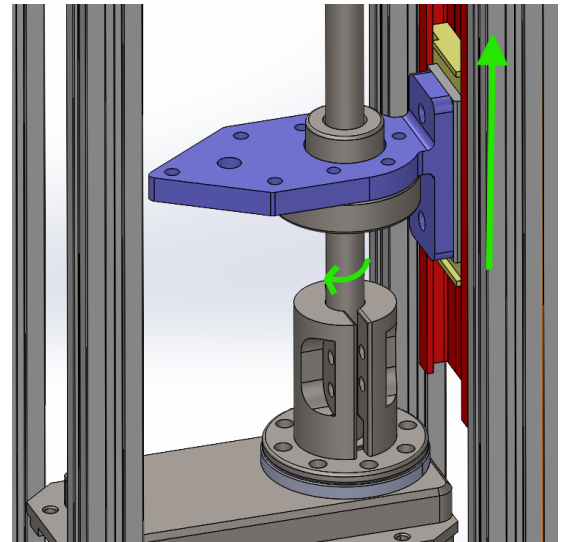
(b) Notre système vis-écrou avec la glissière accrochée au support
