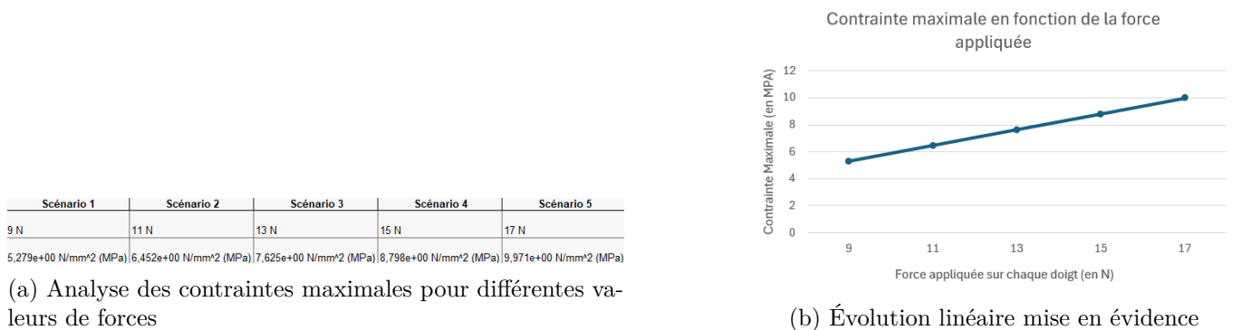
FIGURE IV.3 – Analyse des contraintes maximales et mise en évidence de l'évolution linéaire, traduisant le fait que l'on reste globalement dans le domaine élastique
