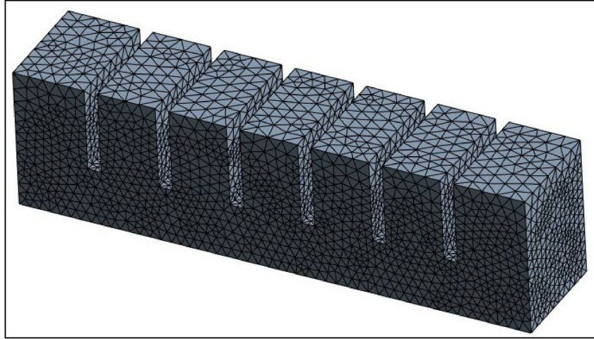
FIGURE II.8 – Représentation du maillage du doigt [?]
