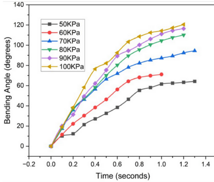
FIGURE II.10 – Angle parcouru suivant la pression exercée lors de l’expérience [?]
