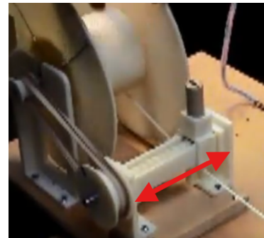
(b) Illustration du mécanisme d'enroulement [?]
