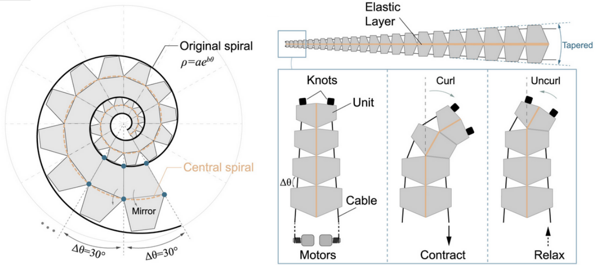
FIGURE II.3 – Spiral logarithmique du préhenseur [?]
