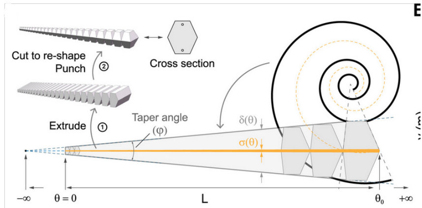
FIGURE III.2 – Construction du doigt en "dépliant" la spirale logarithmique [?]
