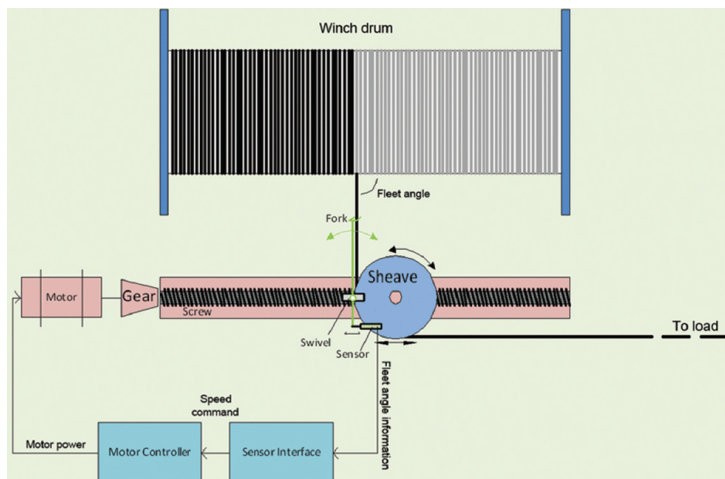
(a) Principe de fonctionnement du système type level wind [?]
