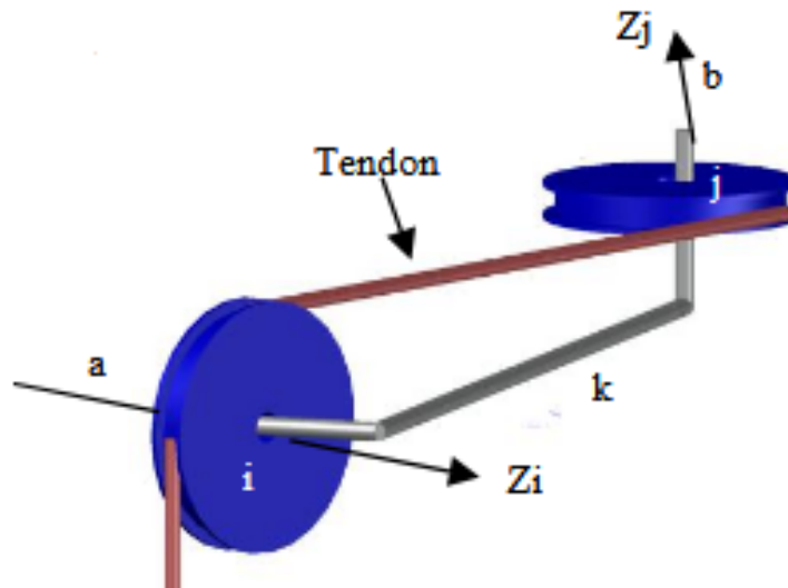
FIGURE II.5 – Tendon à extrémité ouverte [?]
