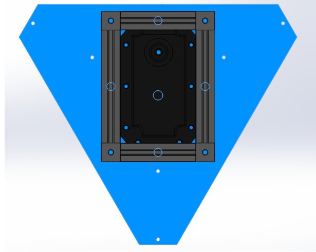
(b) 4 trous de diamètre 4.3 mm dans la base pour fixer les 4 barres
