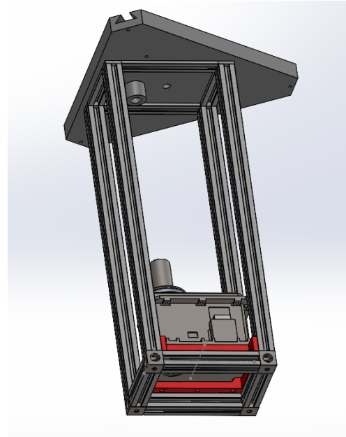
(b) Support assemblé avec la pièce de fixation du moteur (en rouge)
