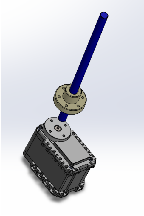
(a) Pièce manquante pour attacher le moteur Dynamixel à la vis mère
