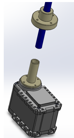
(b) Attache pour la vis et le moteur
