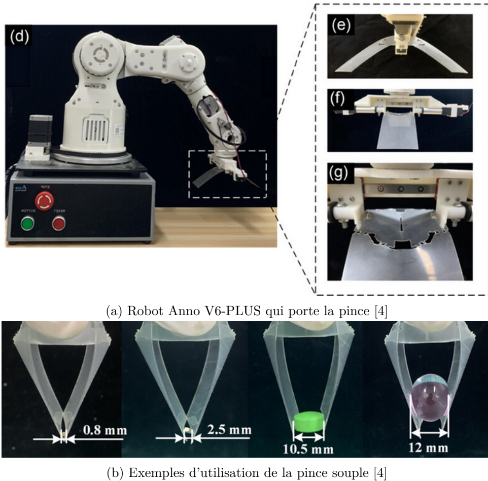
FIGURE II.1 – Illustration de l'étude sur la pince souple
