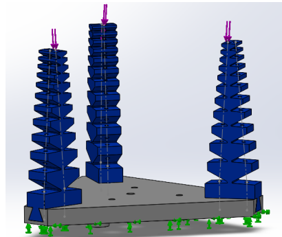
(b) Simulation des forces (en violet) engendrées par les câbles sur l'extrémité des doigts
