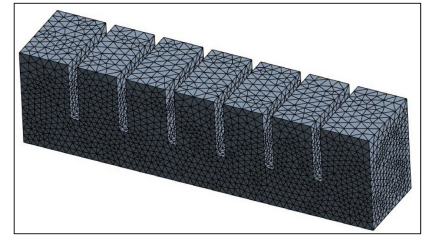
(b) Représentation du maillage du doigt [7]
