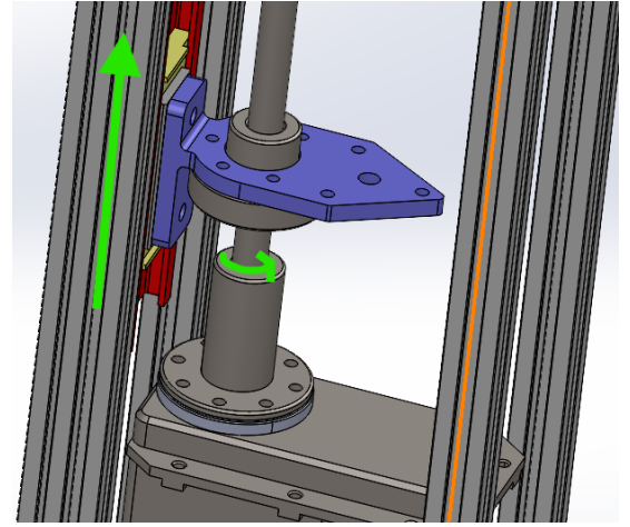
(b) Notre système vis-écrou avec la glissière accrochée au support
