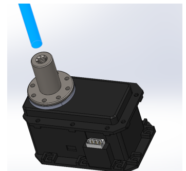
(b) Attache pour la vis mère (en bleue) et le moteur
