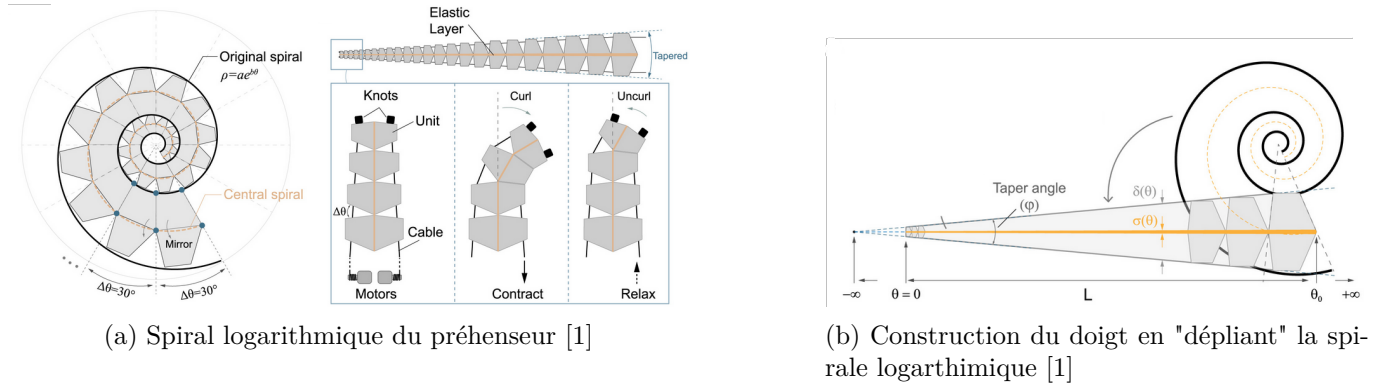
FIGURE I.1 – Conception du doigt
