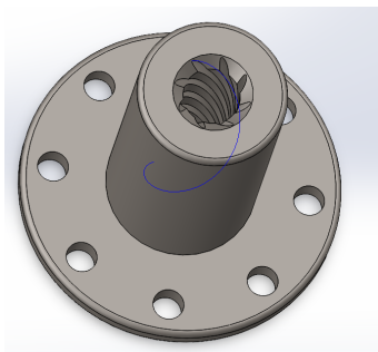
(a) Pièce attachée au moteur et vissée sur la vis mère avec un filetage réaliste
