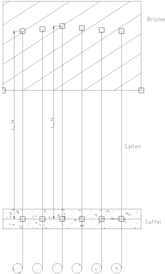
Abbildung 5: Draufsicht des physikalischen Modells mit Saiten-Hebelarmen
