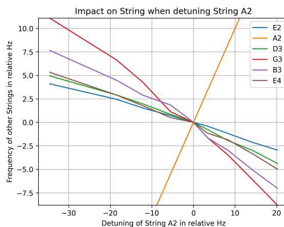
Abbildung 24: Relativer Einfluss der A2 Saite auf die anderen Saiten
