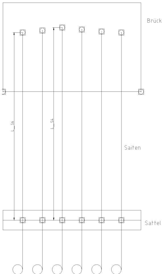
Abbildung 21: Floyd-Rose-Modell Draufsicht
